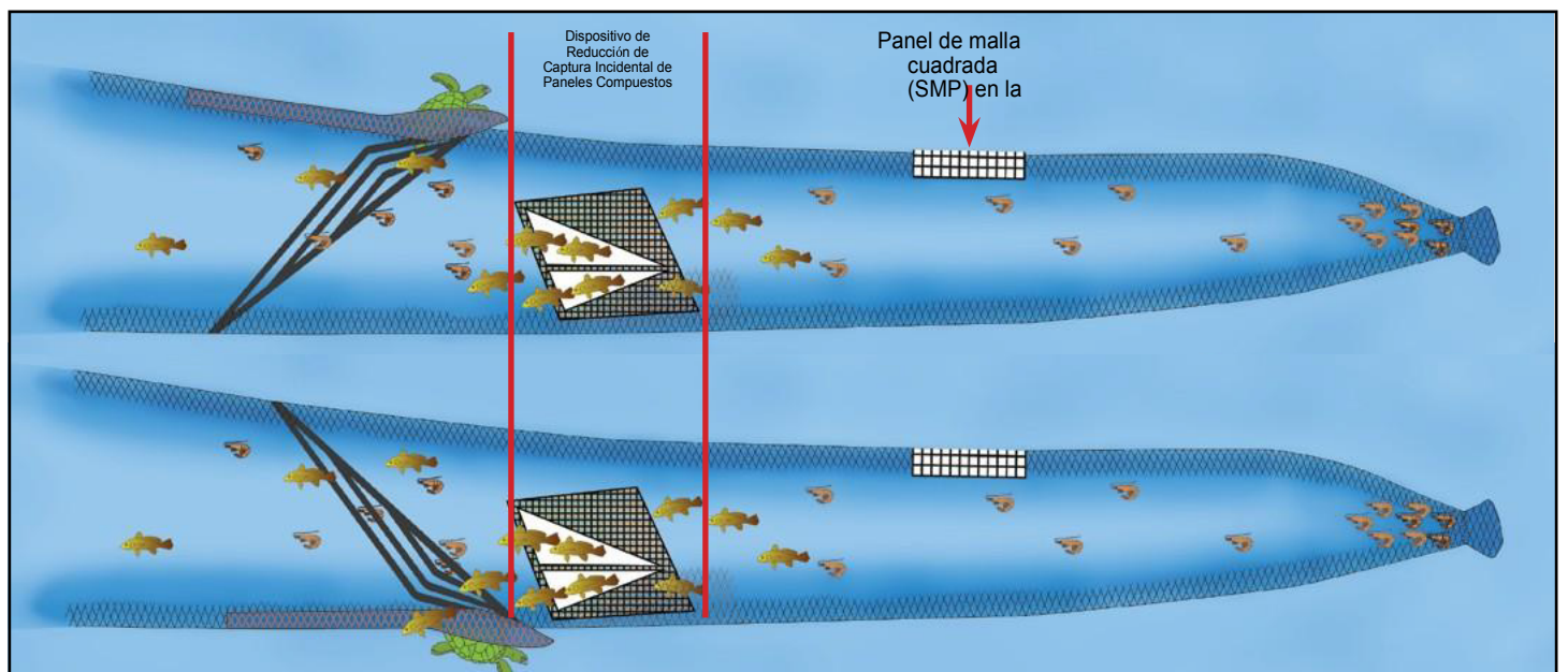
Figura B. Ilustración lateral de un TED de tiro superior y un TED de tiro inferior con Dispositivos de Reducción de Captura Incidentales de Panel Compuesto instalados correctamente en la red de arrastre detrás del TED. Más abajo de la red de arrastre hay un Panel de Malla Cuadrada unido a la parte superior de la red de arrastre.
