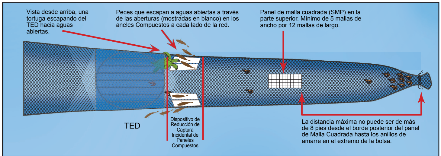
Figura A. Visto desde arriba, una red de arrastre de camarón que ilustra un TED de tiro superior, seguido del Dispositivo de Reducción de Captura Incidentales de Panel Compuesto (con aberturas a cada lado de la red de arrastre), un Panel de Malla Cuadrada (SMP) en la parte superior de la red de arrastre y el copo.
