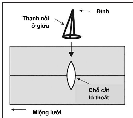
Hình E: Hình minh họa lọc cá kiểu mắt cá đang được lắp đặt vào đọt lưới.
