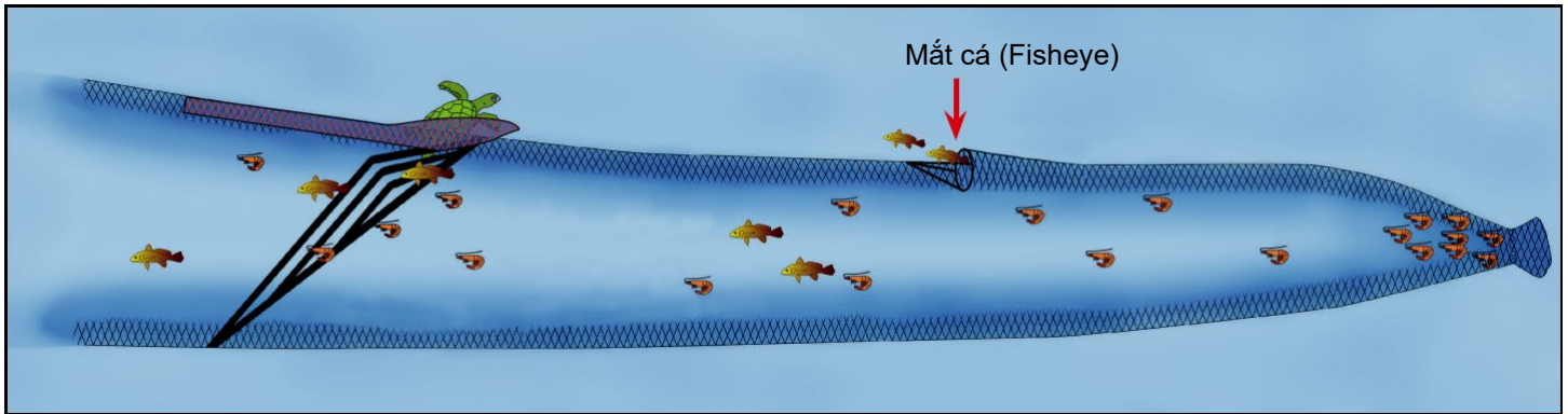
Hình A: Hình ảnh của một khung Lọc Cá (BRD) kiểu mắt cá nằm ở đọt lưới phía sau Thiết bị lọc rùa (TED).
